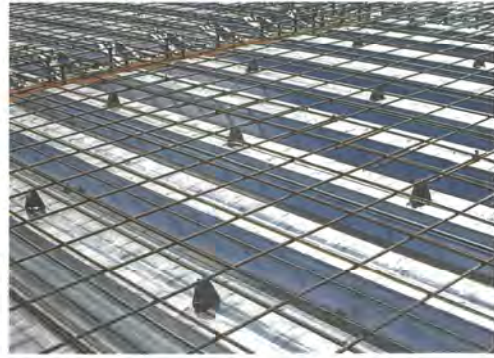
アストンが開発したスペーサー。上部のへばみに鉄筋をはめて固定する
